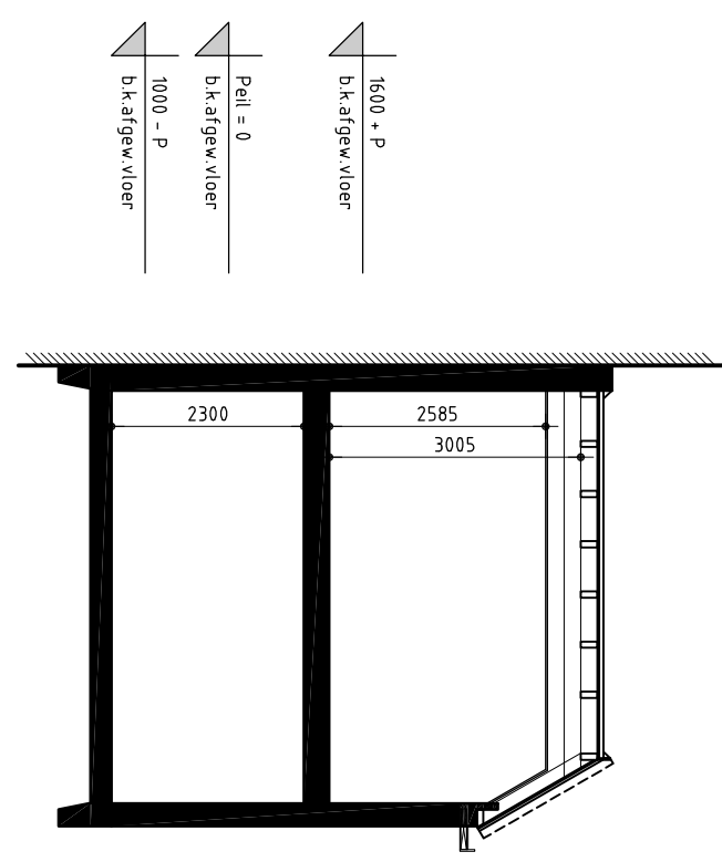
DOORSNEDDE C - C
